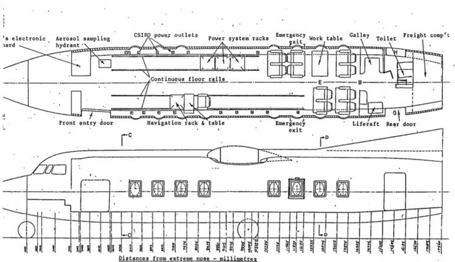
FIG. 3 CSIRO F 27 CABIN LAYOUT
